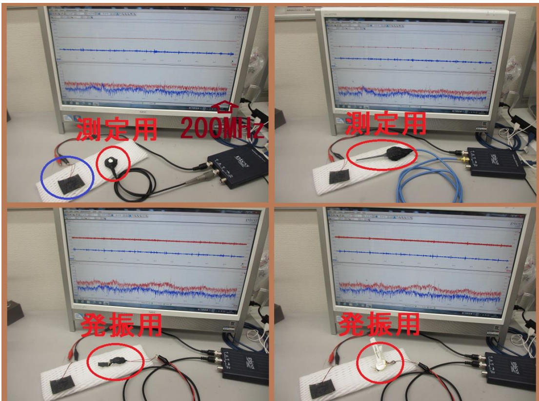
超音波プローブの伝搬特性テスト
