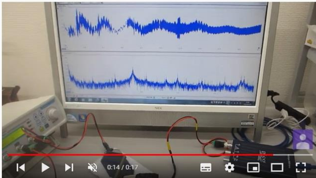
超音波の発振制御による最適化実験（表面弾性波の相互作用）
