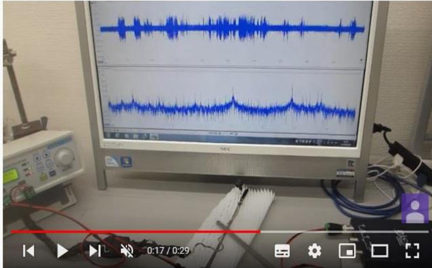
新しい超音波プローブを利用した超音波発振制御実験（超音波の送受信テスト）
