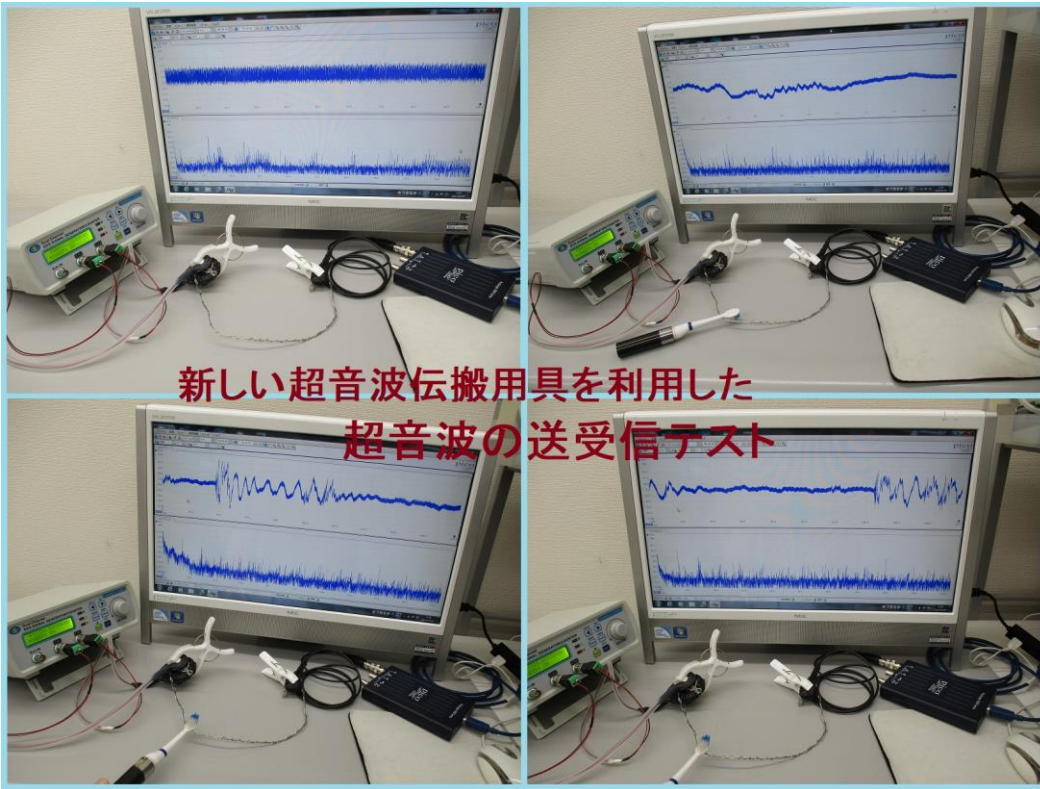
カッターの刃を伝搬する超音波
