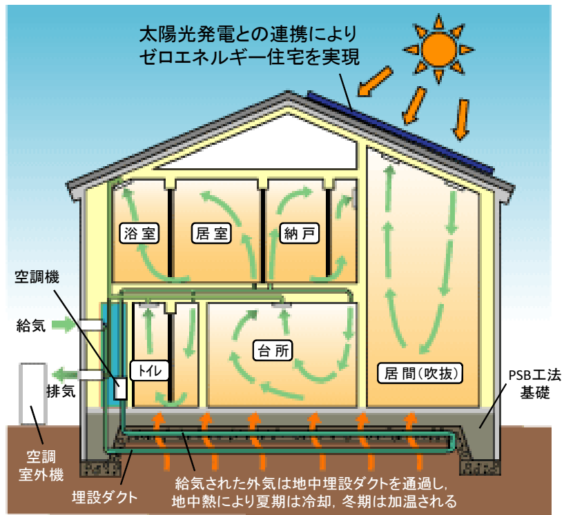
【図1】 HAS ver. 9 (地熱利用) の概念図
