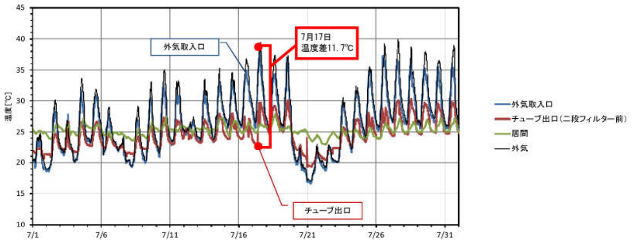
前橋宿泊体験展示場温度グラフ
