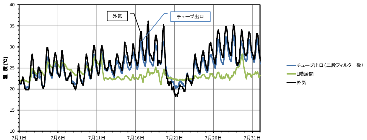
前橋宿泊体験展示場温度グラフ
